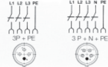
Настенная розетка
