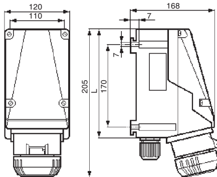
настенная розетка
