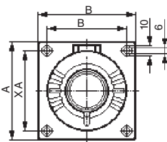
муфта
