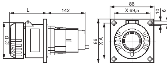
муфта
