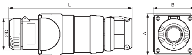
муфта
