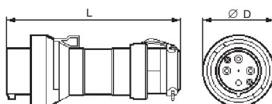
штекер
