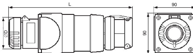
штекер
